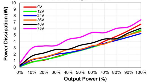
CQB50W8-36S12 Pd Vs Po @25 Deg. C
