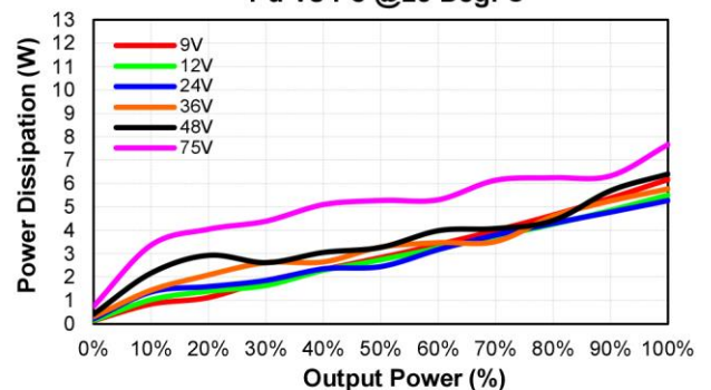
CQB50W8-36S28 Pd Vs Po @25 Deg. C
