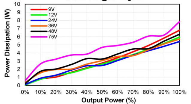
CQB50W8-36S15 Pd Vs Po @25 Deg. C
