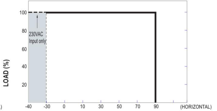
T_{case} (°C)
