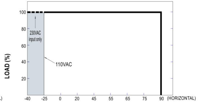
T_{case} (°C)
